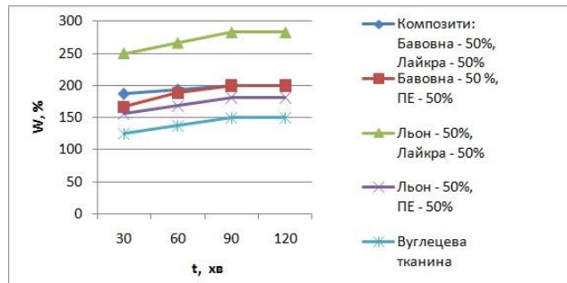
Рисунок 3 – Вплив сировинного складу нетканої основи композиційно ранового покриття на вологості
