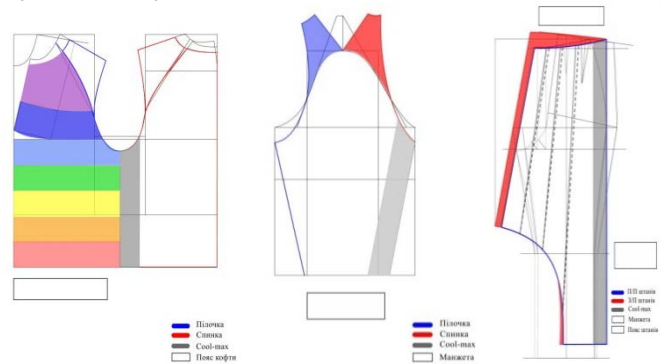
Рис. 4. Кресленки МК основи кофти, рукава реглан та штанів-афгані
