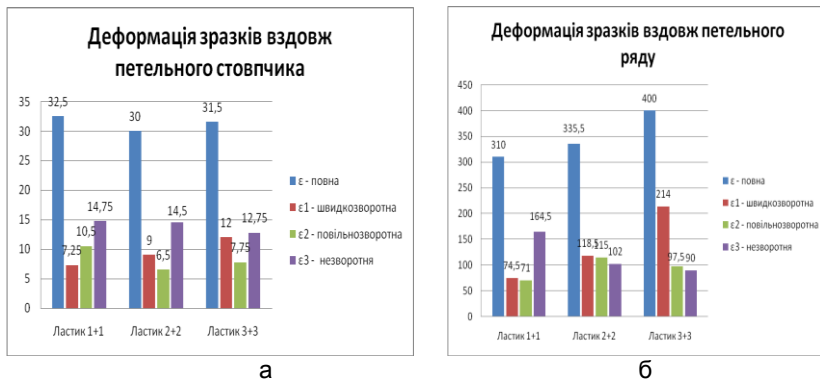
Рис. 2. Деформації зразків ластик 1+1, 2+2, 3+3 вздовж петельного стовпчика (а) та вздовж петельного ряду (б)
