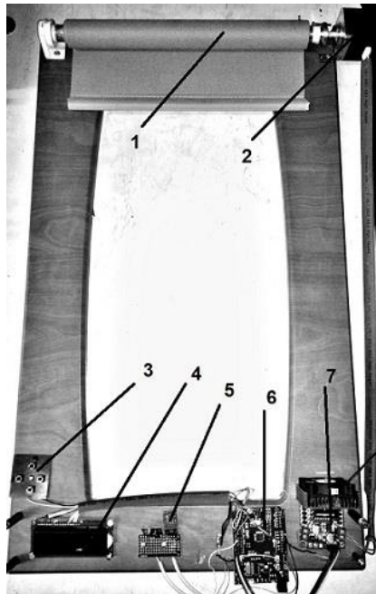
Рис. 2. Загальний вигляд лабораторного стенду: 1) ролети; 2) кроковий двигун; 3) меню; 4) дисплей; 5) датчик температури та вологості; 6) контролер Arduino Uno; 7) драйвер крокового двигуна
