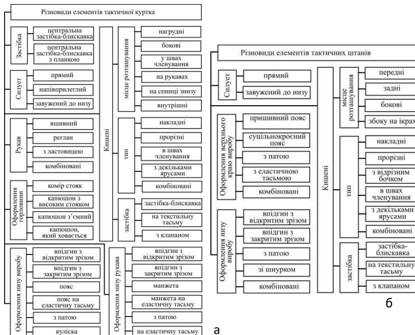
Рис.1. Узагальнення конструктивно-композиційних елементів тактичної: а – куртки, б – штанів
