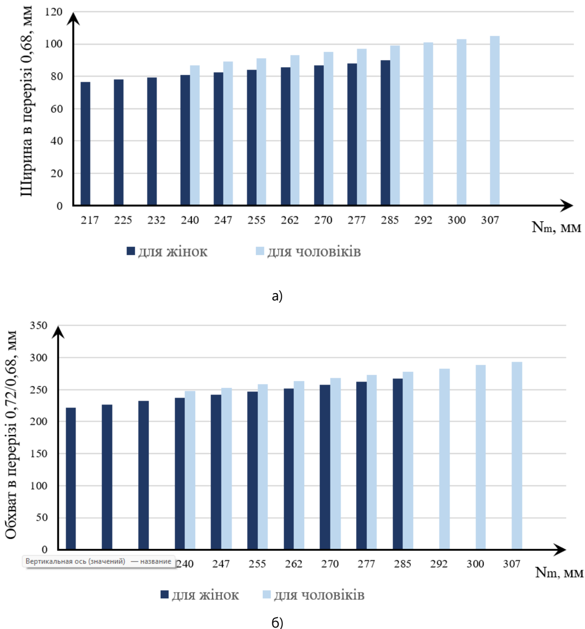
Рис. 3. Діаграма відмінності між широтними та обхватними параметрами колодок для чоловічого та жіночого спеціального взуття при однаковому розмірі взуття в метричній системі
