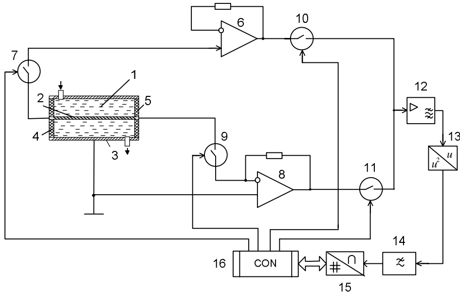
Рис. 1. Функціональна схема виміру активного опору високоомних рідин 1 – коаксіальна кондуктометрична комірка із внутрішнім електродом 2 і зовнішнім електродом 3; 4, 5 – ізоляційні шайби; 6 – повторювач напруги; 7, 9, 10, 11 – комутаційні ключі; 8 – перетворювач струму в напругу; 12 – вибіркового підсилювач; 13 – квадратичний перетворювач; 14 – фільтр нижніх частот; 15 – аналого-цифровий перетворювач; 16 – мікроконтролер.
