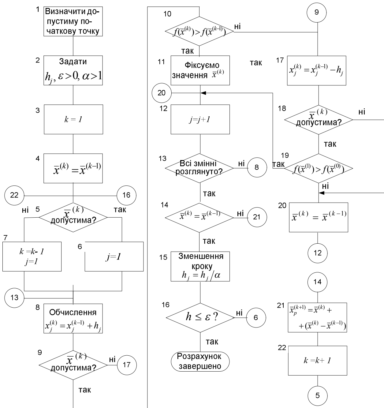
Рис. 1. Алгоритм модифікованого методу Хука-Дживса
