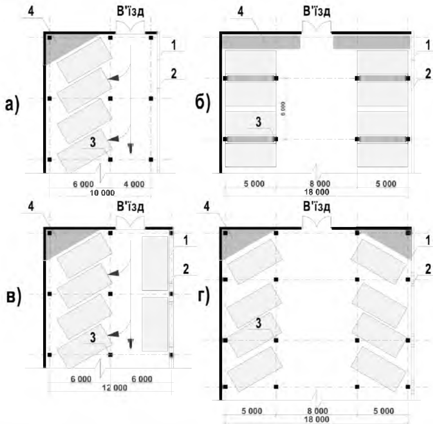
Рис.4. Схема розміщення автомобілів при манежному зберіганні: а), в) – у цегляних одноповерхових будівлях із додатковим перекриттям; б), г) – у каркасних одноповерхових та багатоповерхових будівлях із додатковими перекриттями. 1 – між прогінна стіна у одноповерхових будівлях; 2 - зовнішня стіна у багатоповерхових будівлях; 3 – додаткові колони для обпирання додаткових перекриттів; 4 – простір, що не використовується
