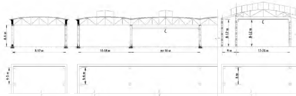
Рис.1. Характерні конструктивні схеми одноповерхових промислових будівель
