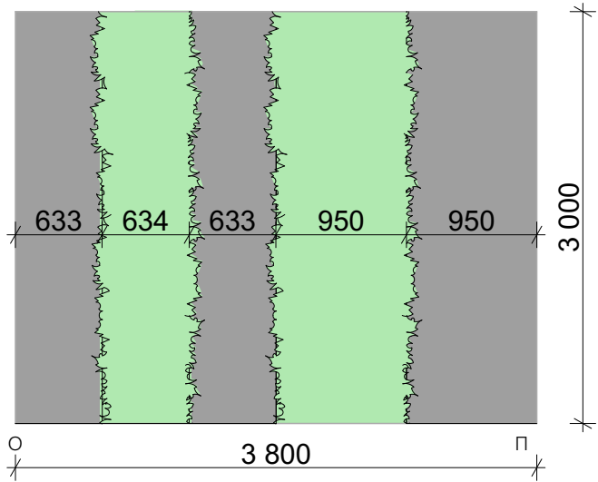
Розгортка О-П 1:50
