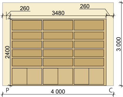
Розгортка P-C 1:80
