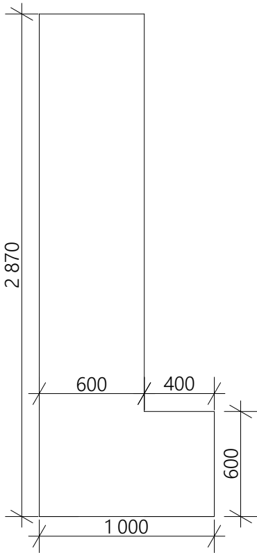
План 1:30
