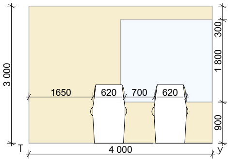
Розгортка T-Y 1:80
