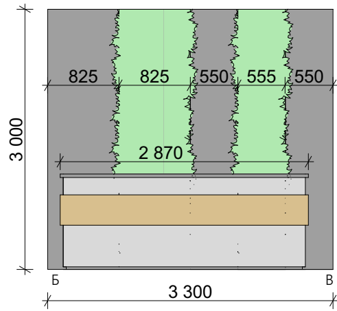
Розгортка Б-В 1:60
