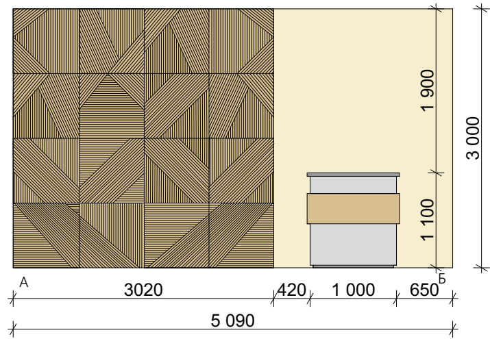
Розгортка А-Б 1:60
