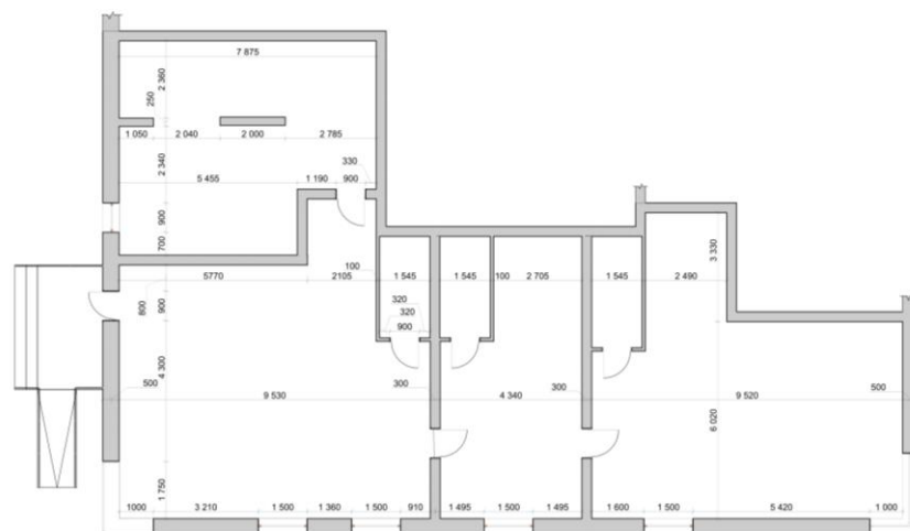
Рис.2.1. Обмірний план
