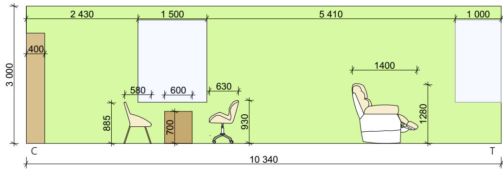
Розгортка C-T 1:80
