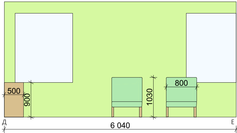
Розгортка Д-Е 1:60
