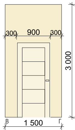
Розгортка В-Г 1:60
