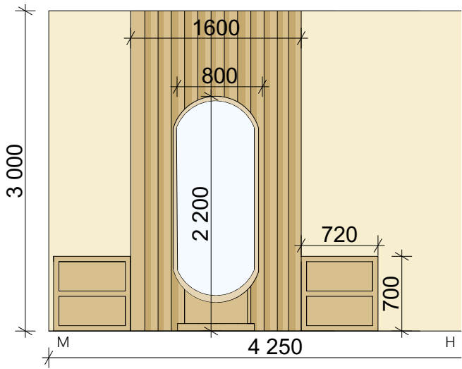
Розгортка М-Н 1:50
