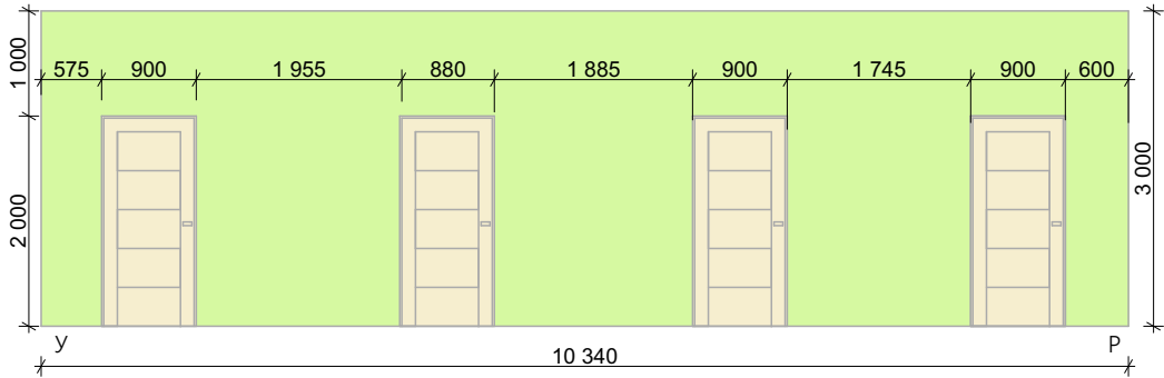
Розгортка Y-P 1:80
