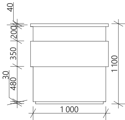
Бічний вид 1:30
