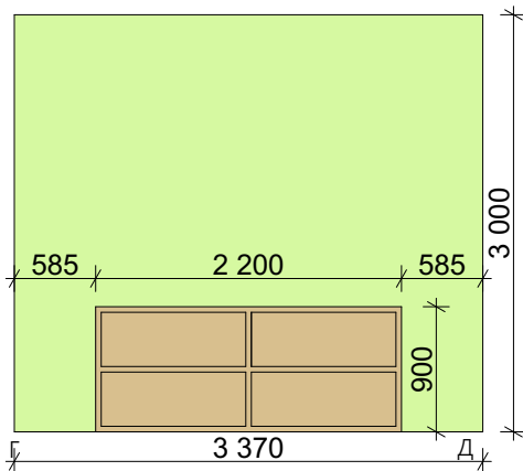
Розгортка Г-Д
