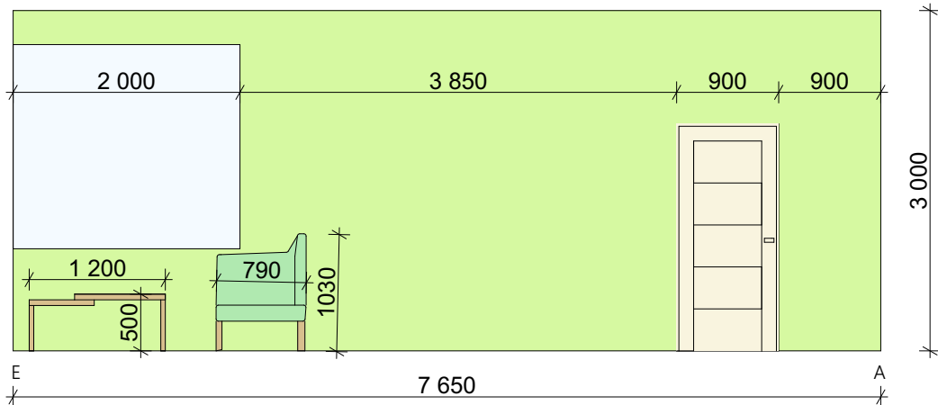
Розгортка Е-А 1:60
