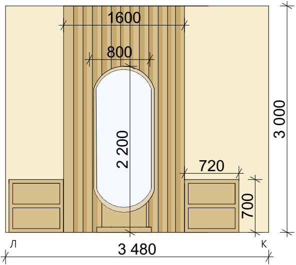
Розгортка Л-К 1:50
