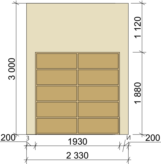
Розгортка З-И 1:50
