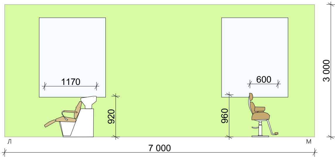
Розгортка Л-М 1:50
