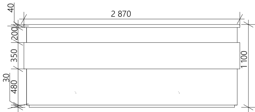
Фронтальний вид 1:30
