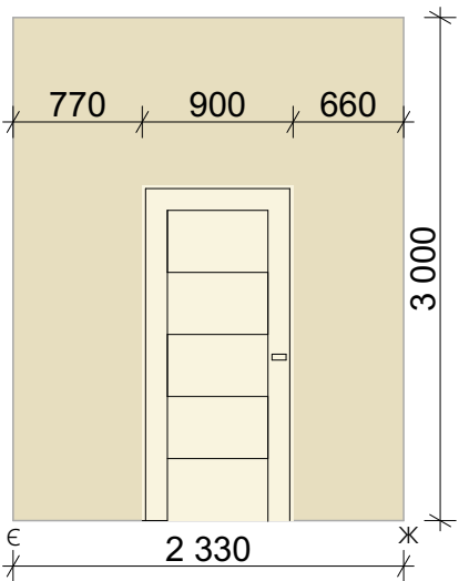
Розгортка Є-Ж 1:50
