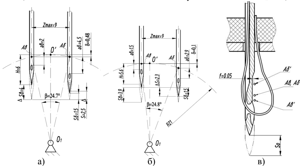
Рисунок 1 – Схеми взаємодії петлеутворюючого органа з «петлями напуску» при близькому Aβ та при віддаленому Aβ' проколах голкою: а) при симетричному розташуванні величини зигзагу Zmax; б) при асиметричному розташуванні величини зигзагу Zmax; в) положення петлеутворюючого органа в площині «петлі-напуску».
